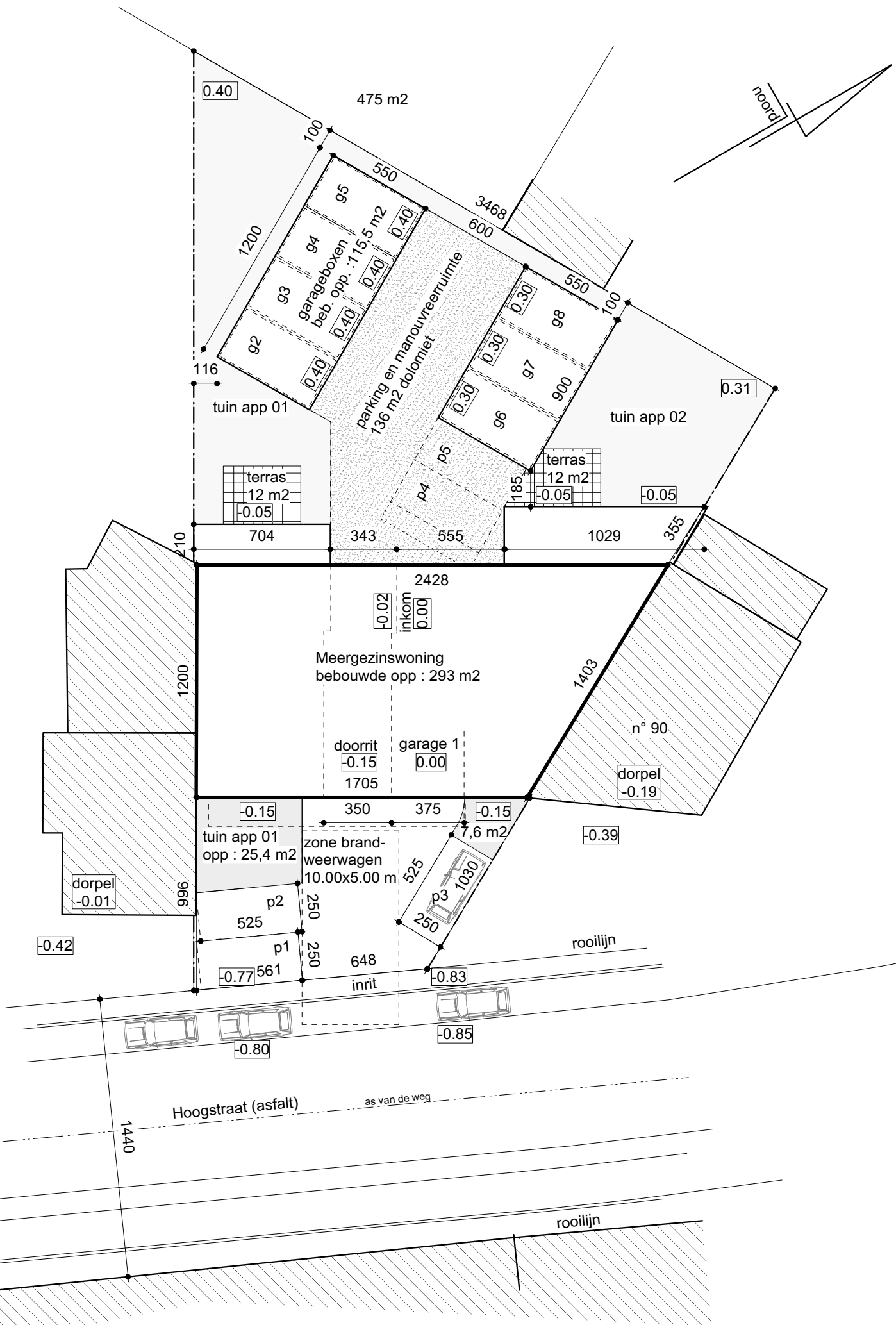
INPLANTINGSPLAN schaal 1/250
