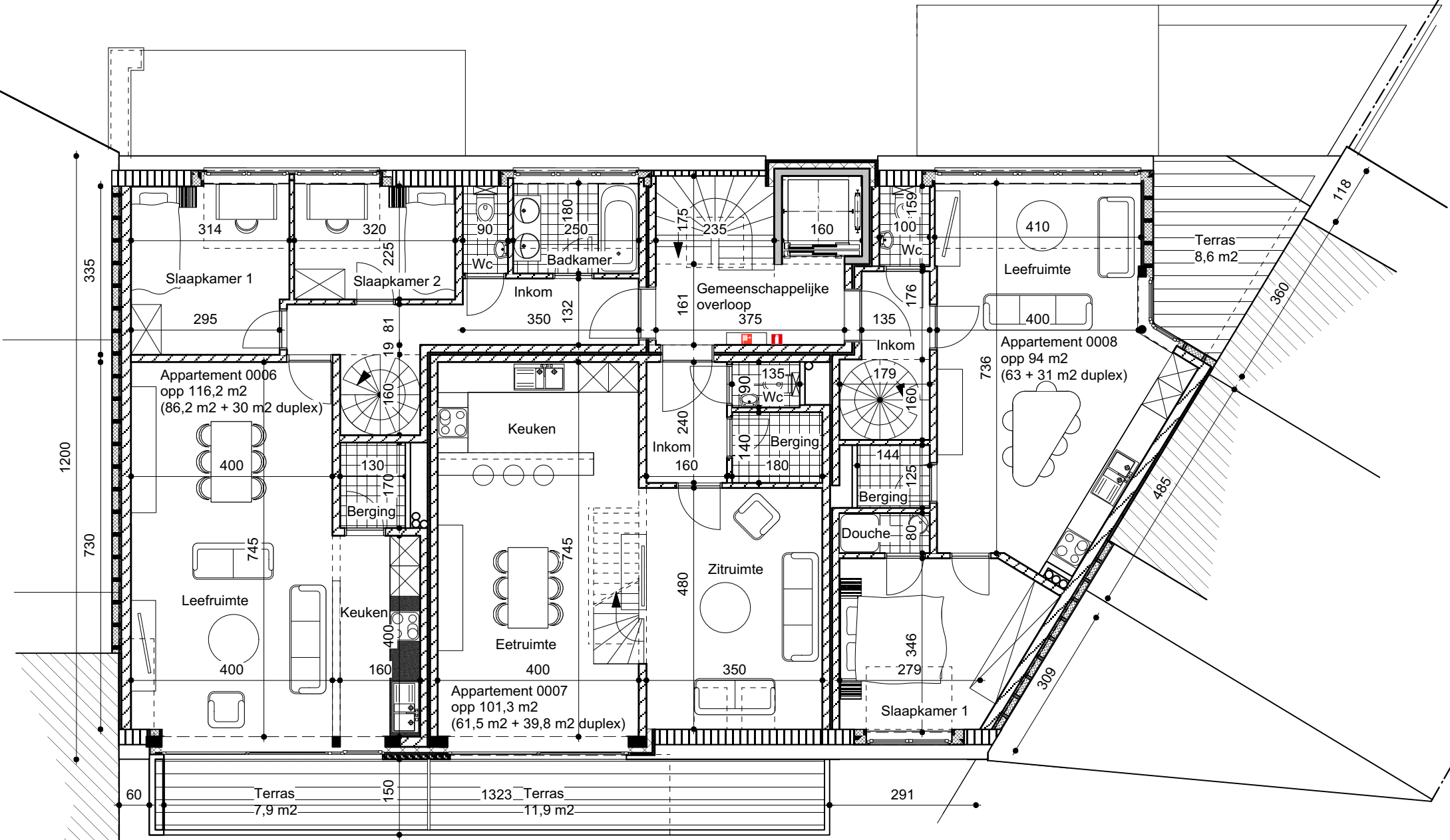
TWEDE VERDIEPING schaal 1/100
