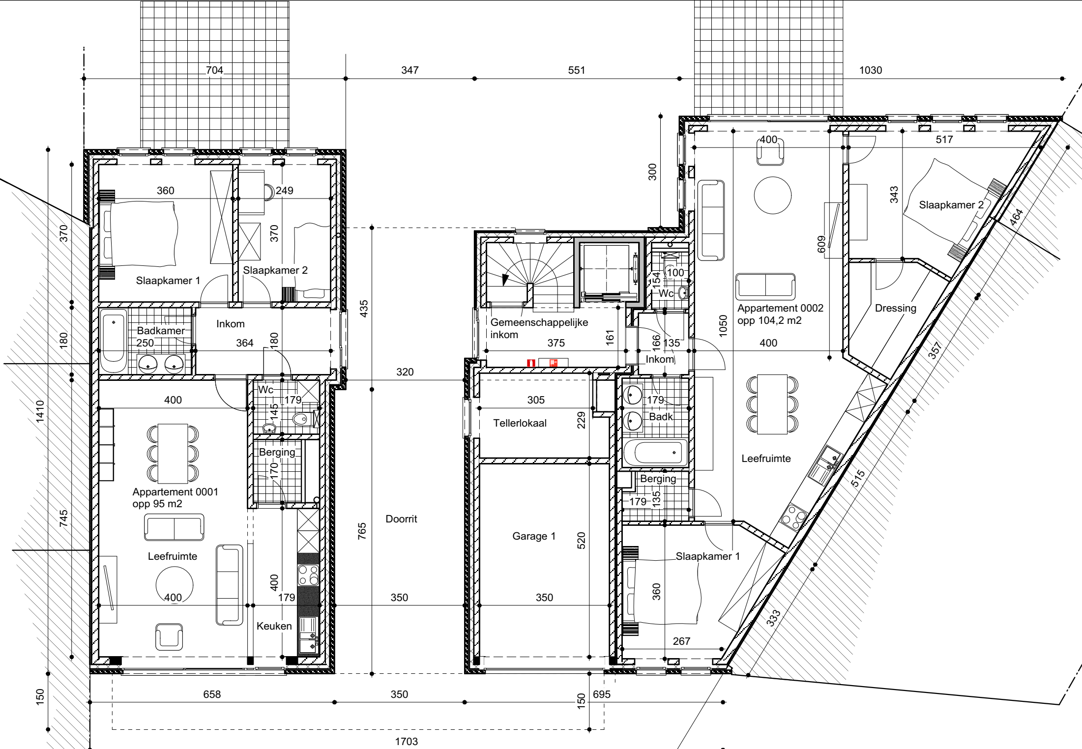
GELIJKVLOERS schaal 1/100
